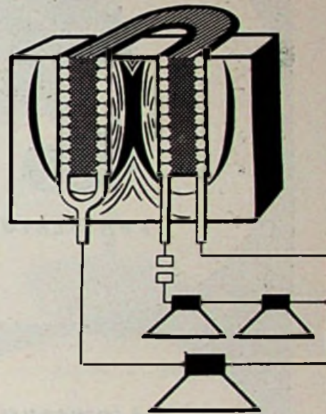
Schematische opbouw van de uitgangstransformator der Blaupunkt radio's, waarbij door de speciale wikkeling het spanningsverlies zeer gering is.
